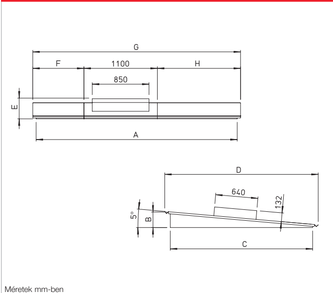
AIR1-AAD RH .../ULM méretek
